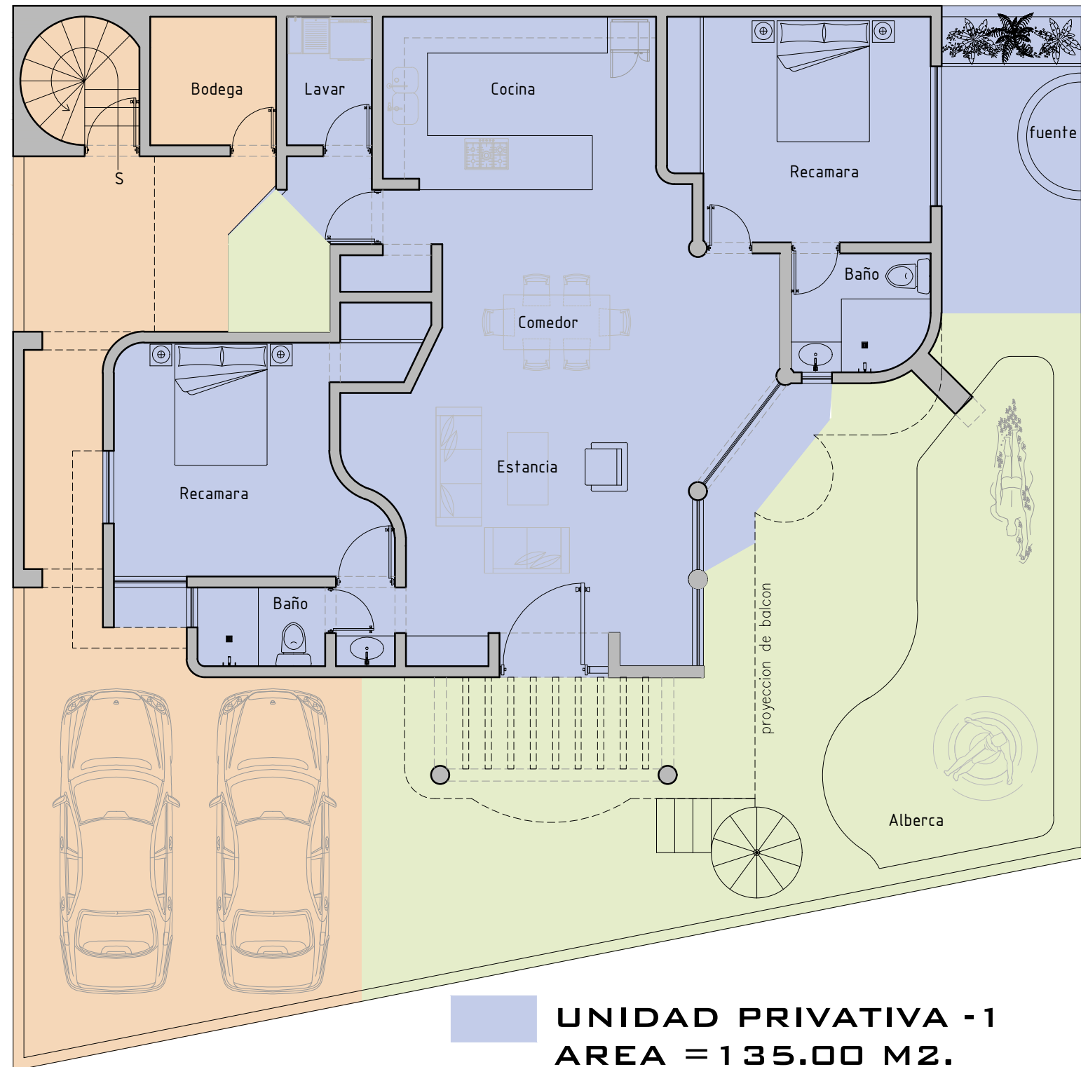
planta B A J A escala 1:100 casa habitacion
