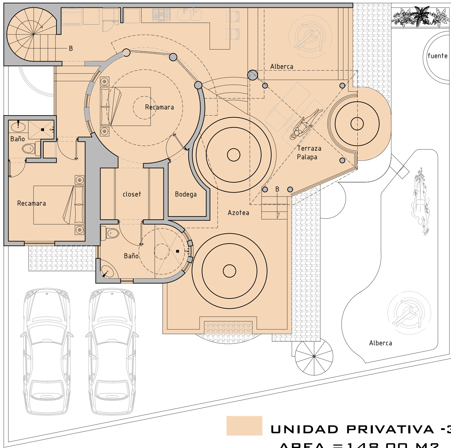
planta SEGUNDO NIVEL escala 1:100 casa habitacion
